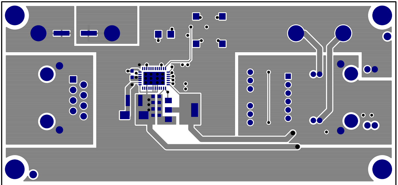
Top Side
