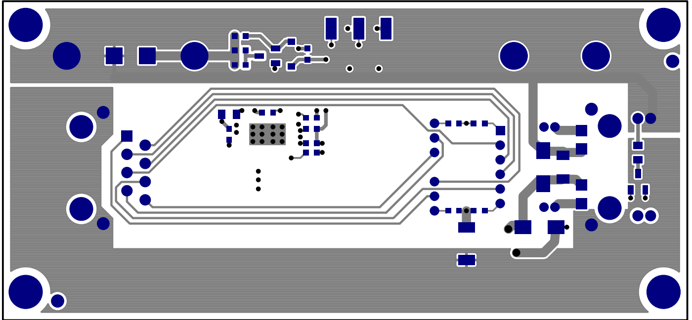
Bottom Side
